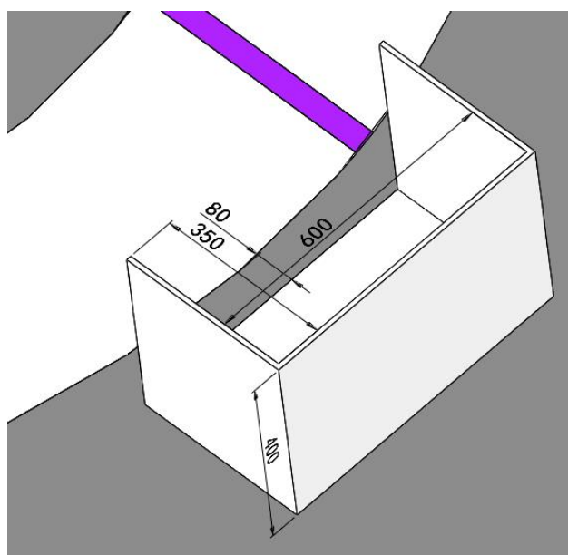
图 8 住户 1 标识尺寸（单位：mm）
