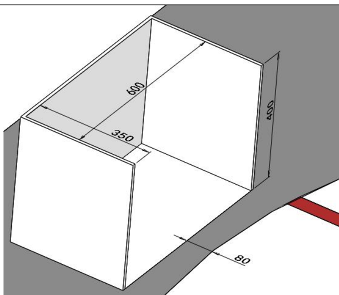
图 9 住户 2 标识尺寸（单位：mm）
