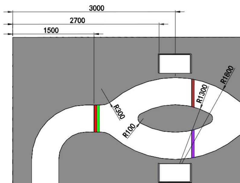
图 5 分岔路尺寸（单位：mm）
