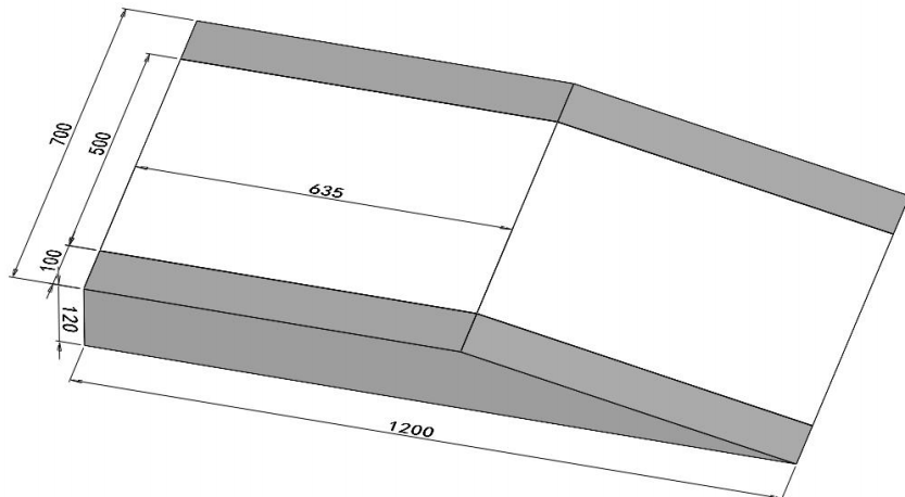
图 6 上斜坡、下高台尺寸（单位：mm）
