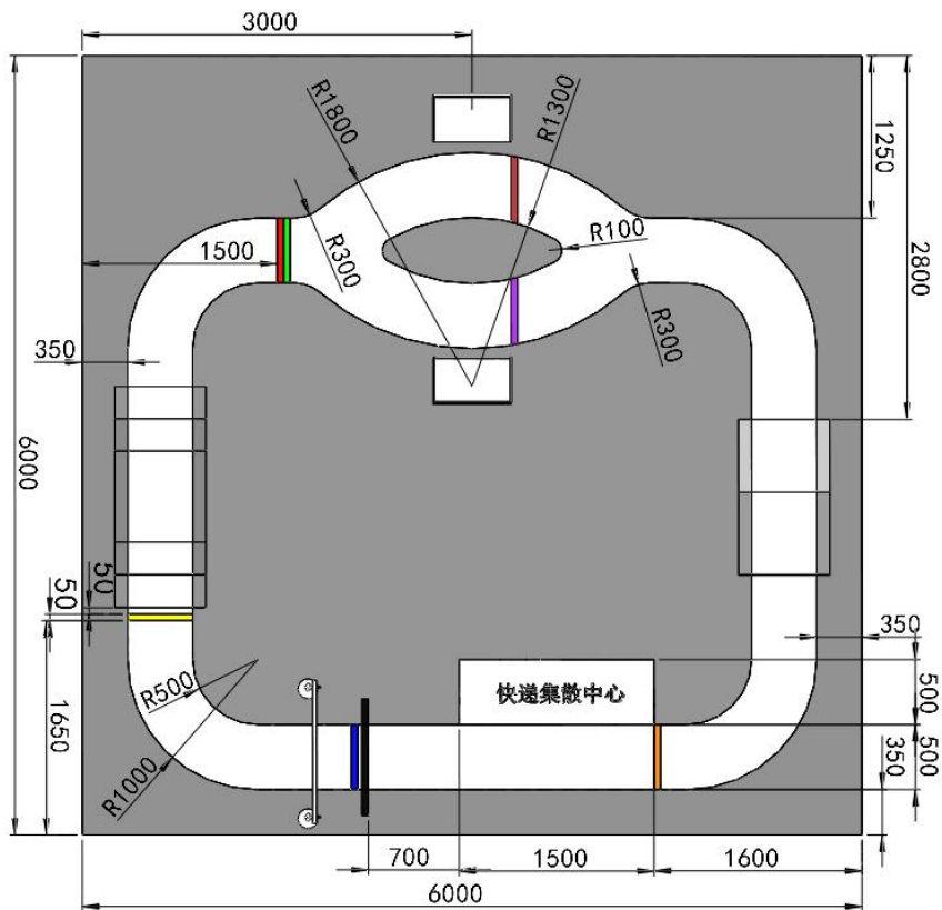
图 1 比赛场地整体尺寸（单位：mm）
