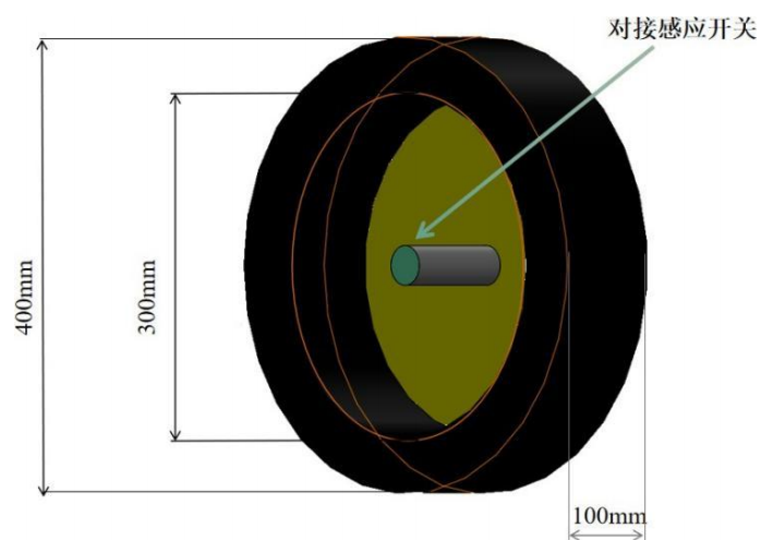
图 3: 星箭对接环结构尺寸示意图
