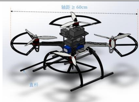
图 4: 无人机结构图
