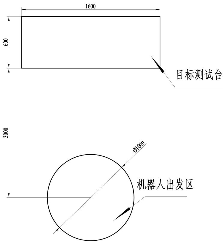
(a) 比赛场地图
