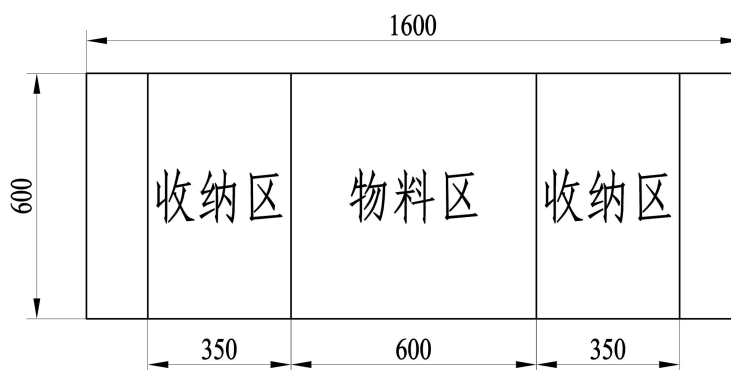
(c) 目标测试台面尺寸图
