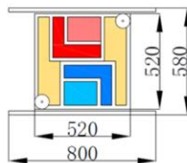
附图 2-3 存储仓
